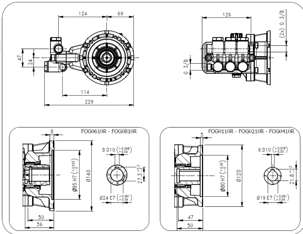
Dimensioni d'ingombro
